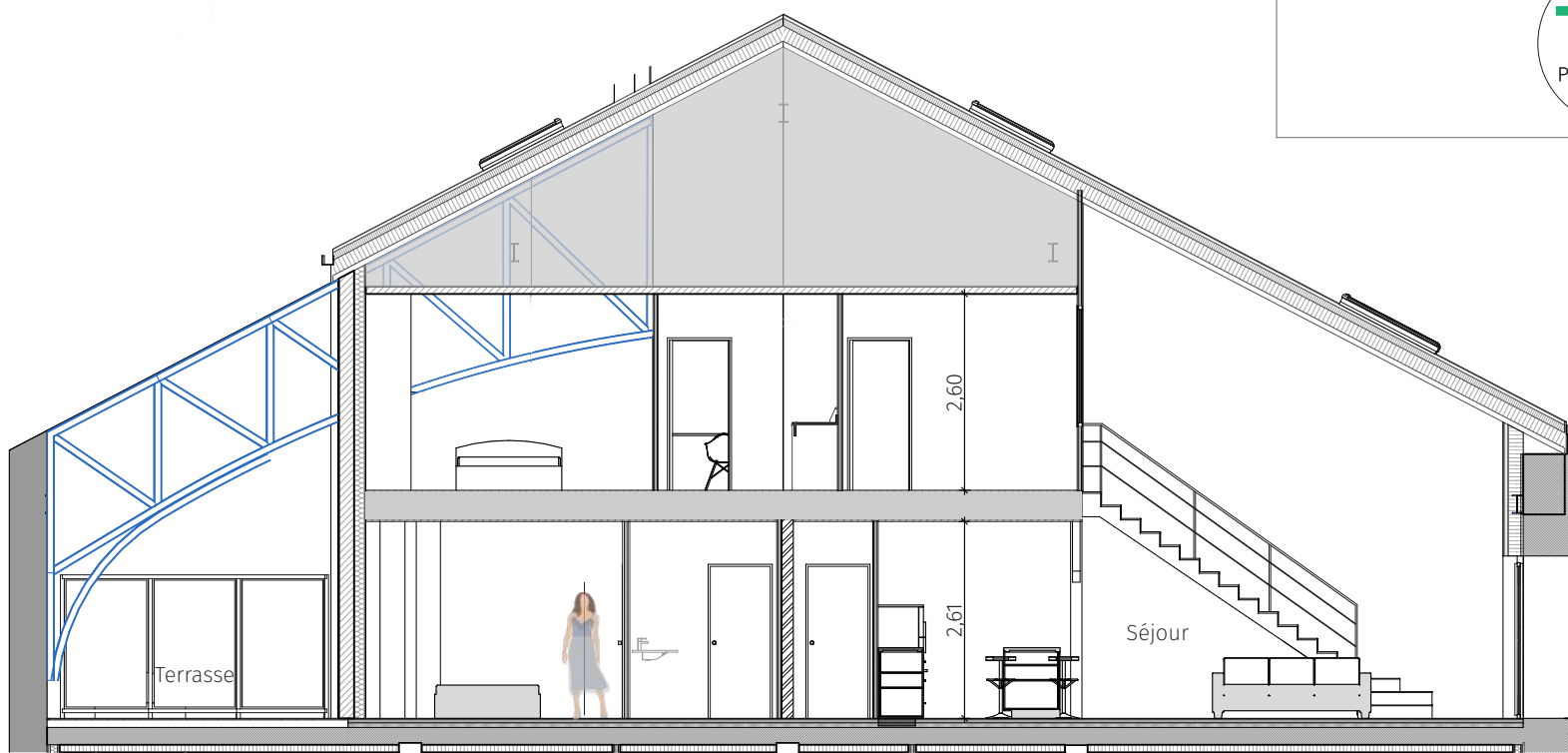
Coupe
